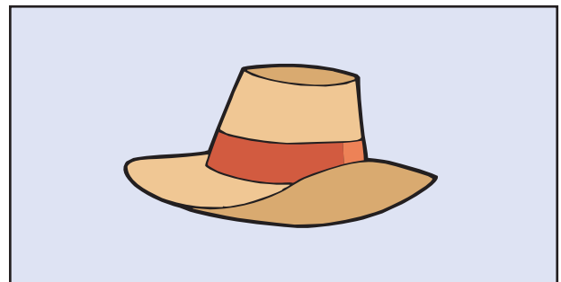
a hat
